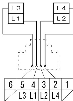
配線図
