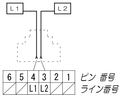
配線図
