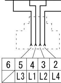
配線図
