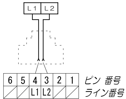
配線図
