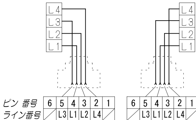
配線図
