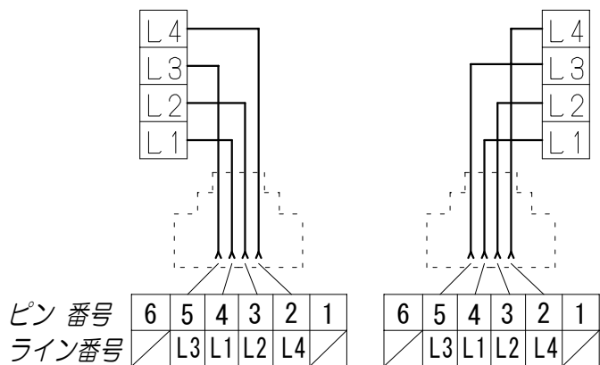
配線図
