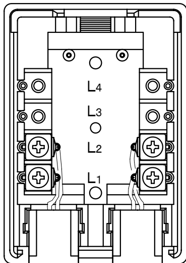
ベース組立図
