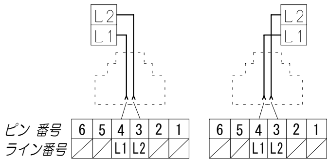
配線図
