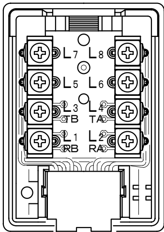
ベース組立図
